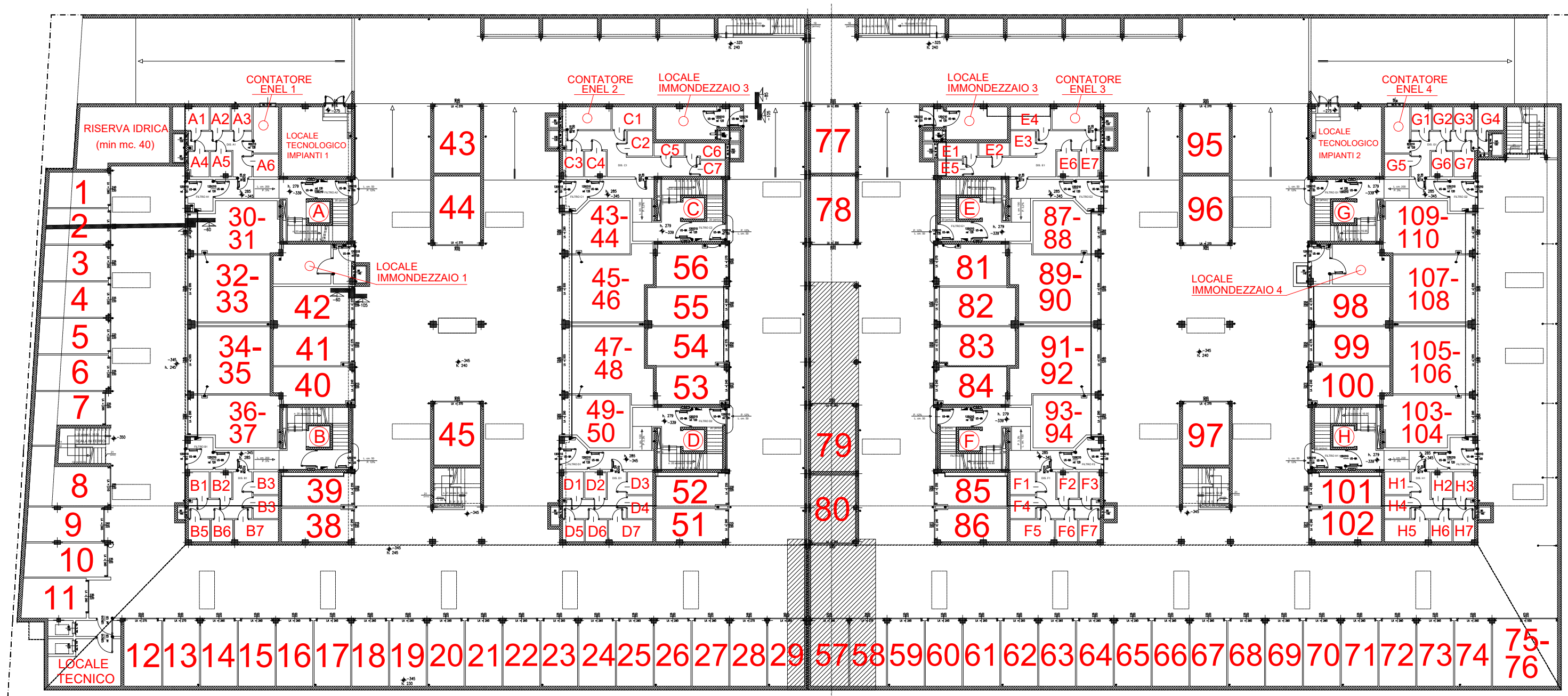
PIANTA PIANO INTERRATO
